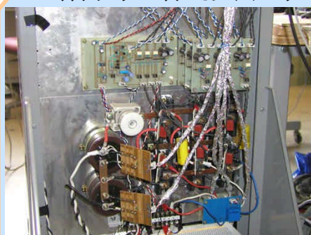
アクティブフィルタ，直接電力制御
