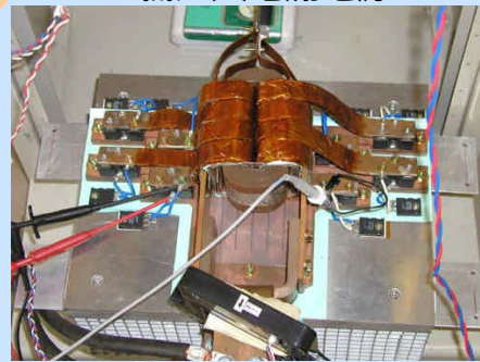
12V-4000A電源
